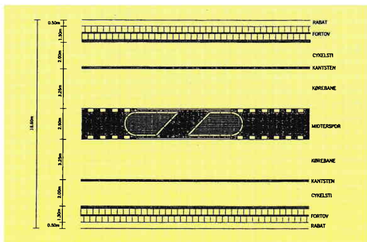
Tværsnit af fremtidens Framlev Korsvej. En lignende konstruktion kendes fra Silkeborgvej gennem Åbyhøj
